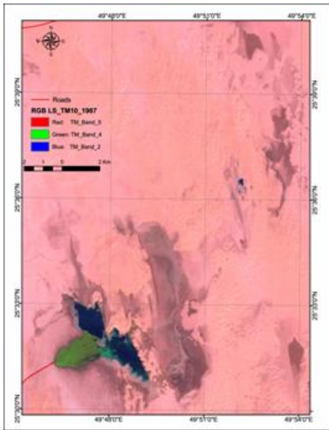
a) Landsat-5 TM, October, 1987
