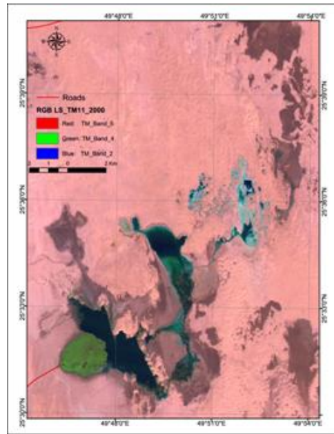
b) Landsat-5 TM, November 2000
